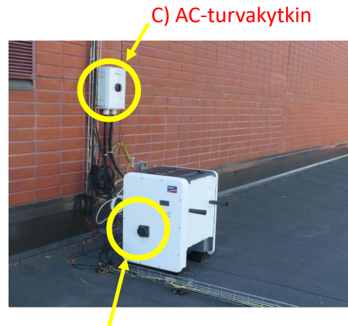
D) DC-turvakytkin
