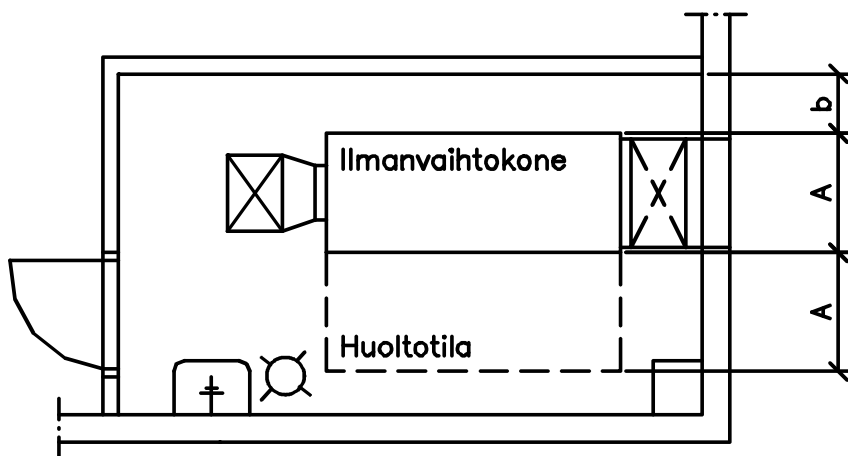
Kuva 5. Koteloidun ilmanvaihtokoneen huoltotilan sijoitus ja mitoitus-esimerkki. A on ilmanvaihtokoneen leveys ja b on 0,4 kertaa ilmanvaihtokoneen korkeus tai vähintään 400 mm.
