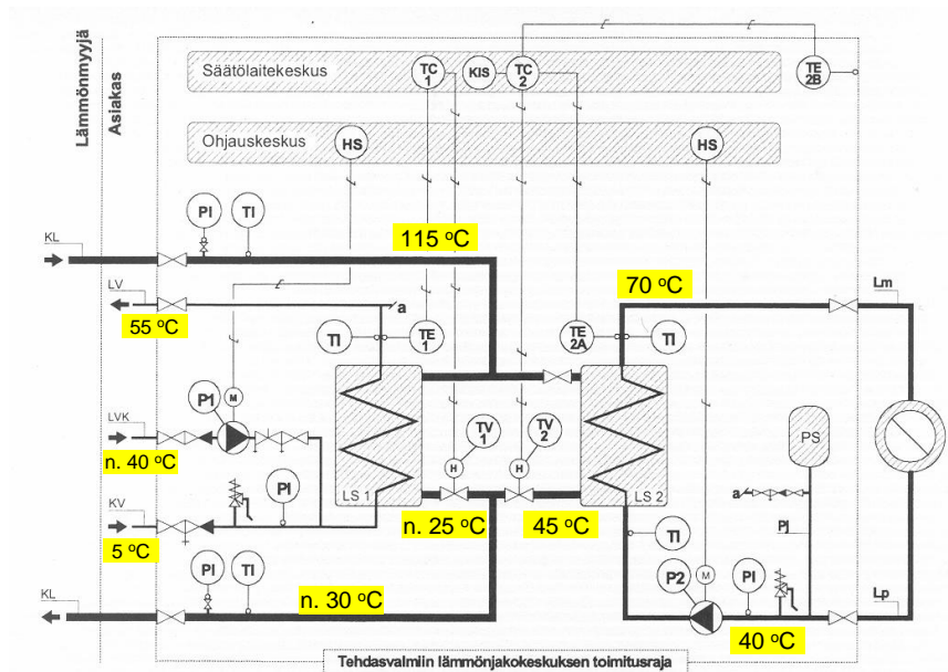
Kuva 3. Kaukolämpökeskuksen lay-out ja eri osien lämpötilat mitoituslaitteessa.
